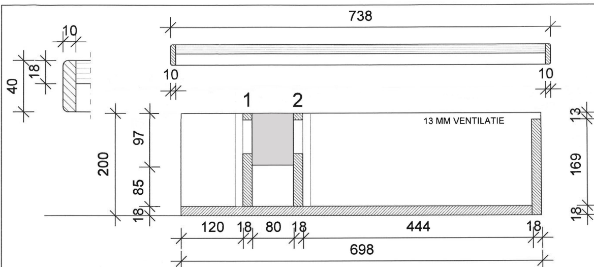
DWARSDOORSNEDE
